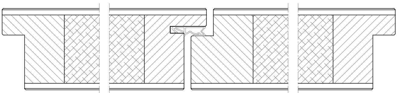
Ausführung 2-flg. / Gangflügel mit Dichtung
